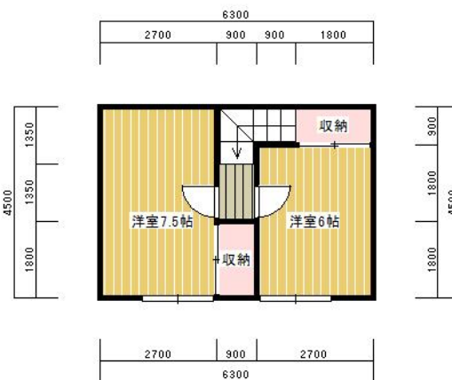
2F
